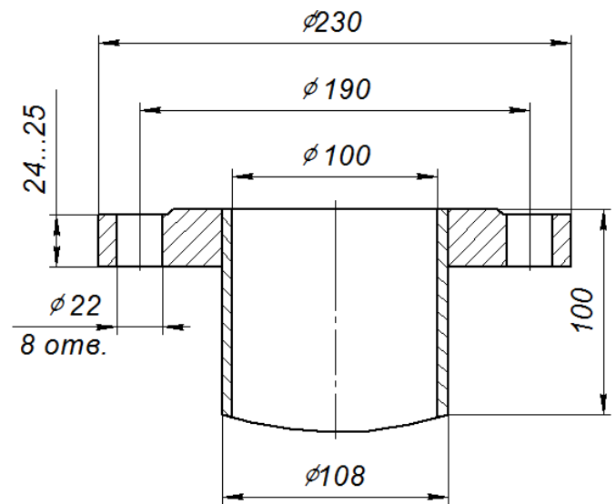
Размеры приварного патрубка на давление 2,5 МПа
