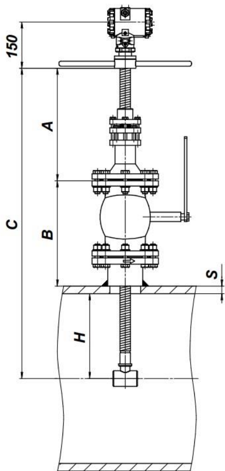
Рисунок 2.4 Вычисление глубины погружения датчика
