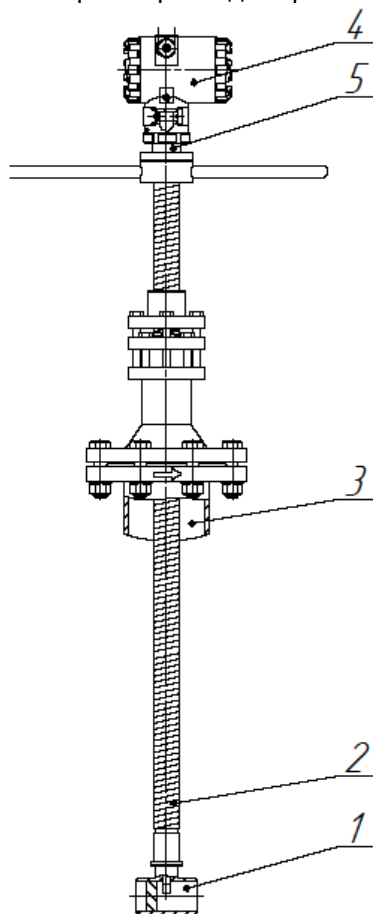
Рисунок 1.1 – Устройство погружных преобразователей расхода
