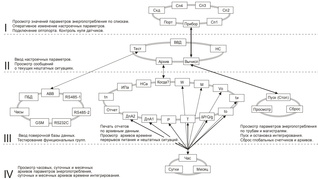
Рисунок 5.1 – Структура меню
