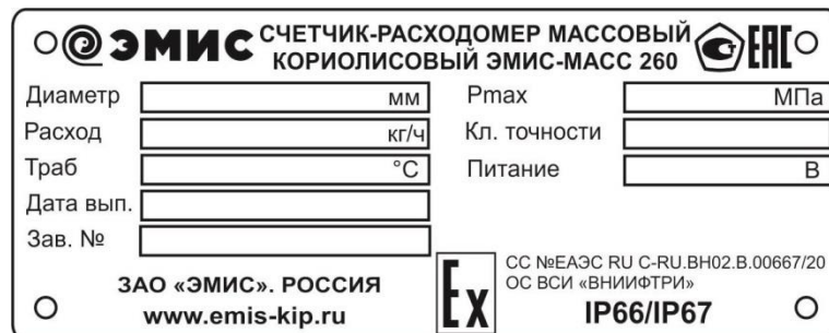
Рисунок 7.1. Шильд электронного блока.
