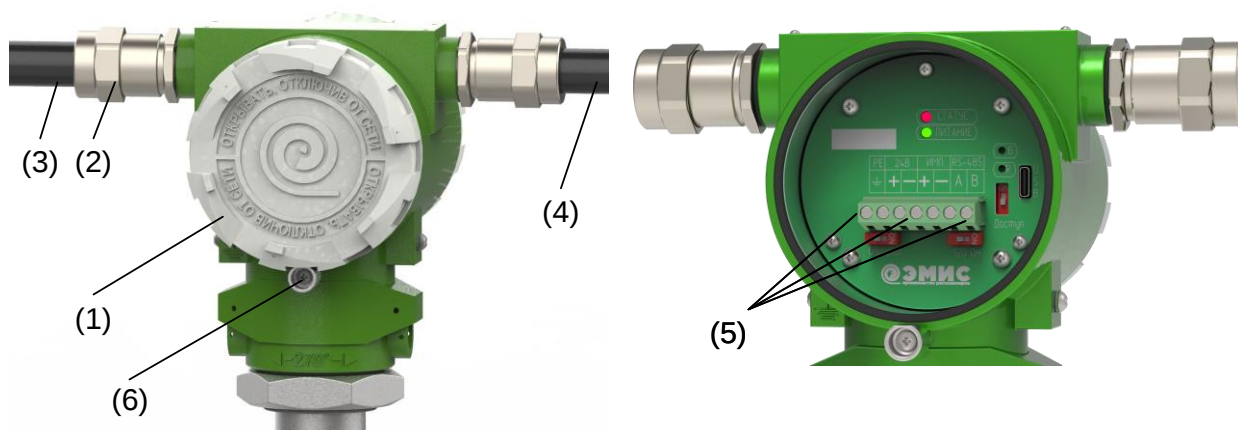
Рисунок 5.4. Электрическое подключение электронного блока.
