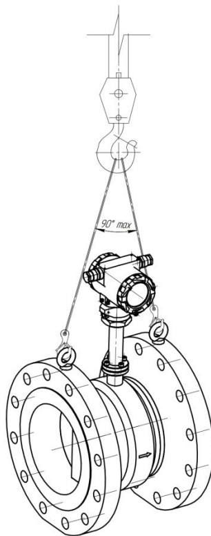
Рисунок 7.1 – Подъем прибора с рым-болтами
