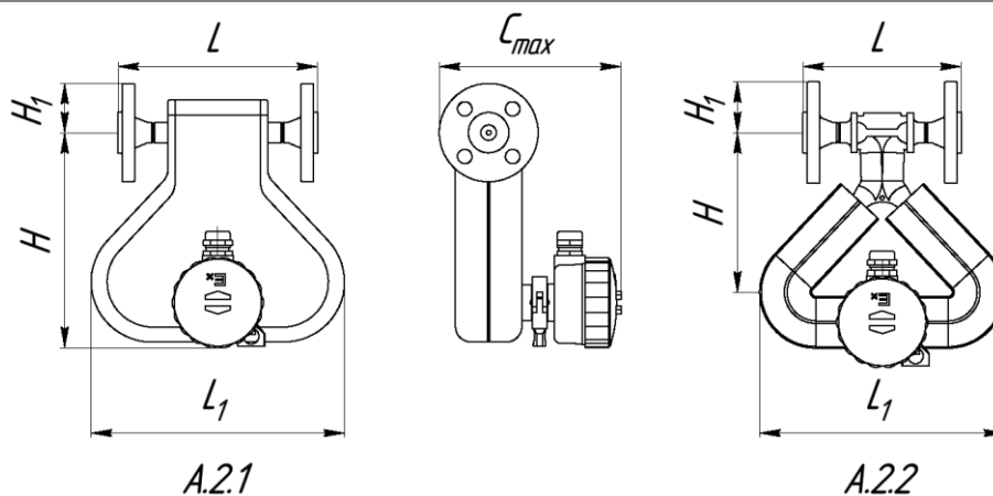
Рисунок А.2 - Габаритные и присоединительные размеры расходомера «ЭМИС-МАСС 260» Ду10-ФРd3, Ду15-ФРd3, Ду10-ФРd6, Ду15-ФРd6
