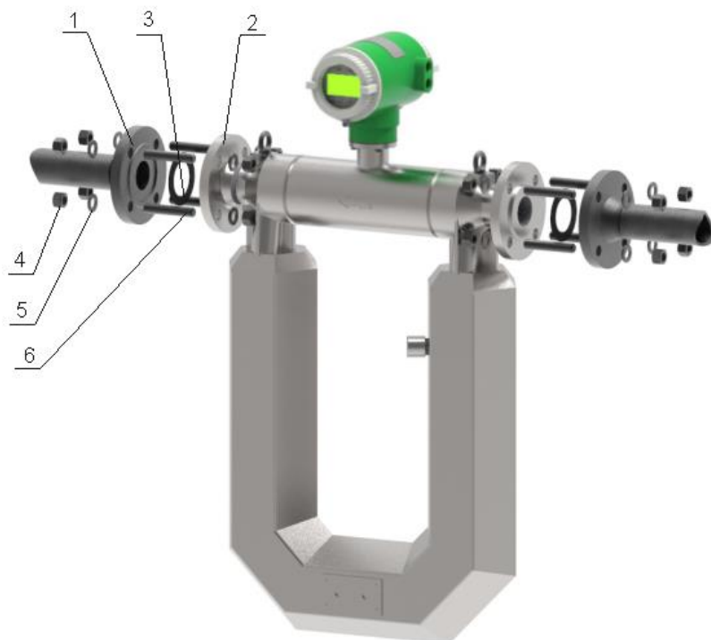
Рисунок 2.6 Установка расходомера «ЭМИС-МАСС 260» на трубопровод
