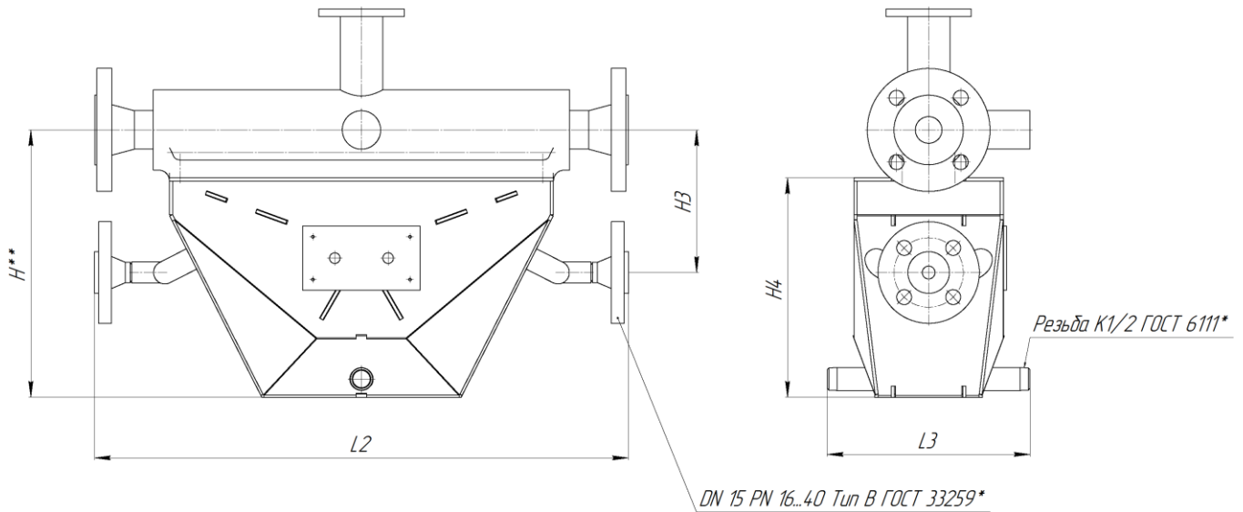
Рисунок А.19 – Размеры рубашки обогрева для типоразмеров 015К и 025К-ФР
