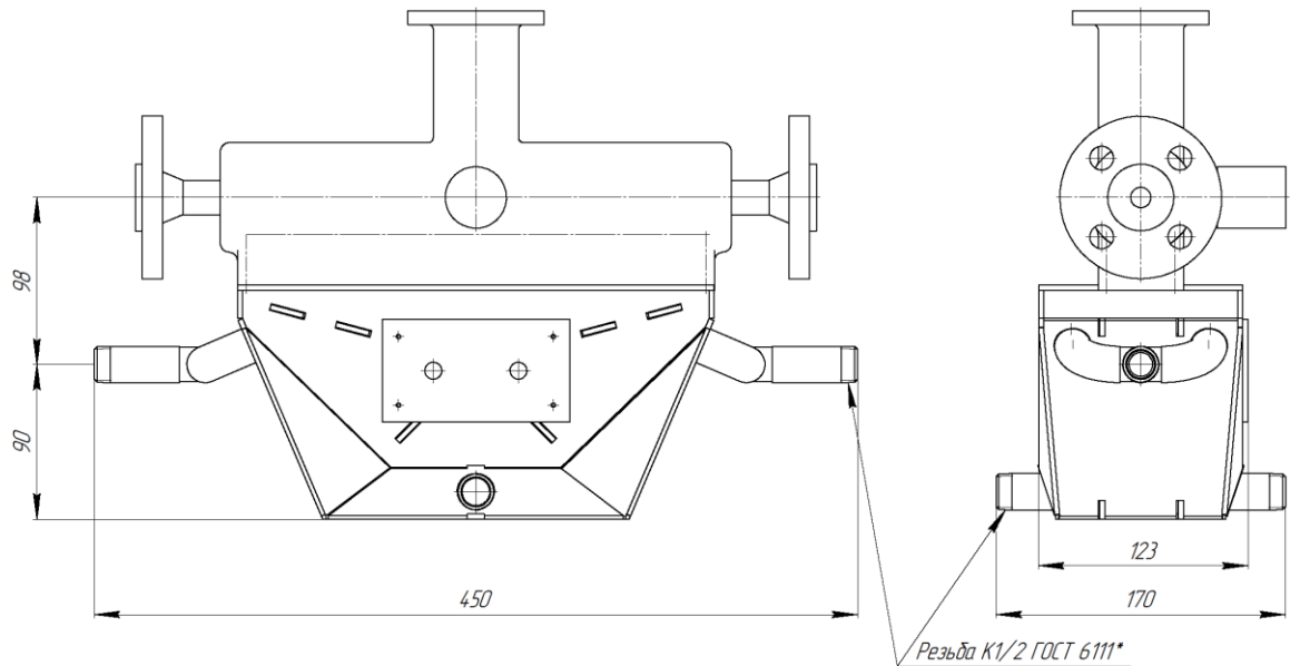
Рисунок А.19 – Размеры рубашки обогрева для типоразмеров 015К и 025К-ФР
