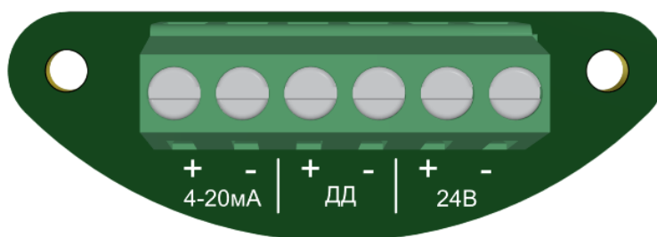
Рисунок 8.2 – Плата коммутации для подключения датчика давления
