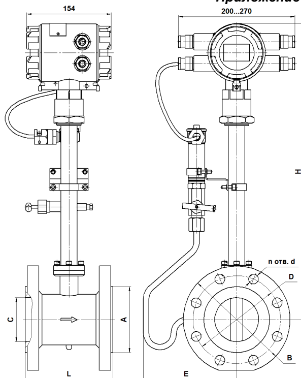
б) с внешним датчиком давления и встроенным термопреобразователем (ВсТД)
