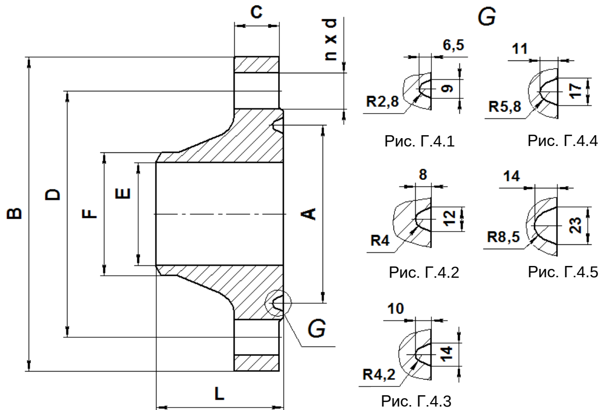
Рисунок Г.4 - Размеры фланцев КМЧ для расходомеров исполнения «Ф1» с давлением 10 - 16 МПа и исполнением уплотнительной поверхности «J»
