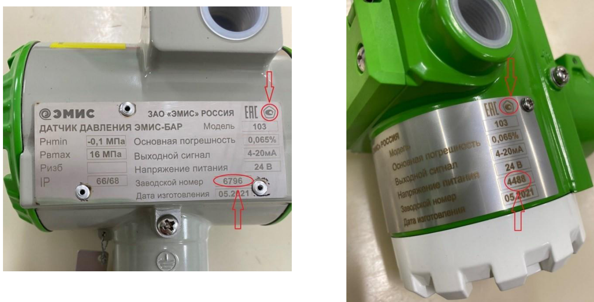
Рисунок 2 – Места расположения заводского номера и знака утверждения типа
