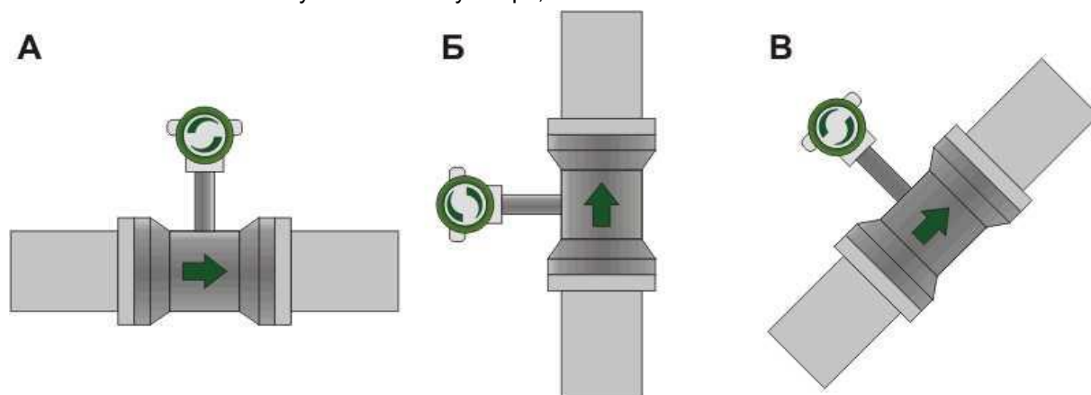
Рисунок 2.2 – Варианты монтажа
