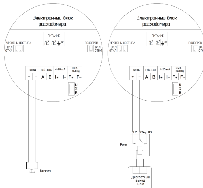
Рисунок 5.9. Схема подключения к входу ЭБ механического выключателя – кнопки (слева) и дискретного выхода через реле (справа).
