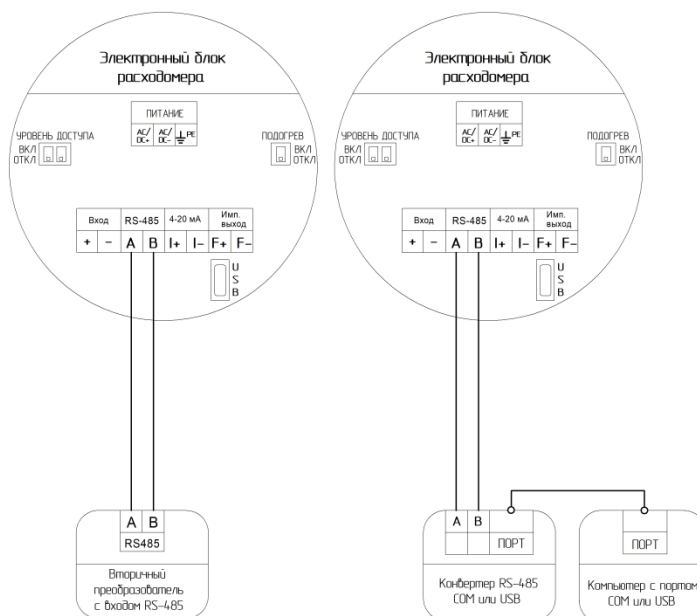
Рисунок 5.6. Схема подключения электронного блока по интерфейсу RS-485 к вторичному преобразователю (слева) и к компьютеру через конвертер (справа).
