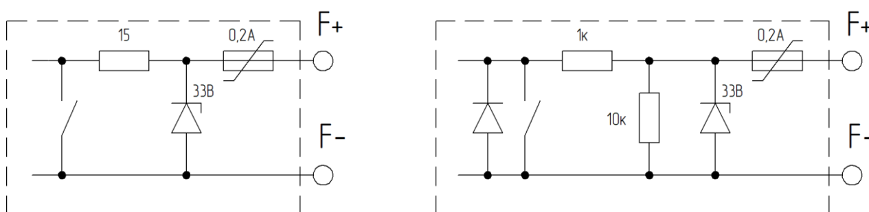
Рисунок 4.2. Схема стандартного (слева) и NAMUR NA01 (справа) частотно-импульсного выхода №1.
