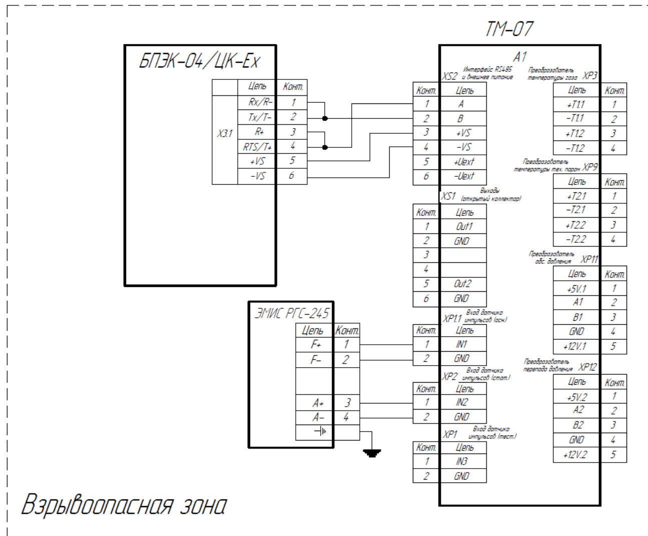
Рисунок В.6 – Схема подключения комплекса учета газа исполнения ЭМИС-ЭСКО 2230-Р-БК, где: ЭМИС-РГС245 – счетчик газа с видом взрывозащиты Exi; TM-07 – Контроллер (в комплекте ДД - датчик давления; ДТ - датчик температуры; ДТ окр.ср.- ДТ окружающей среды (по запросу), ДПД – датчик перепада давления (по запросу); БПЭК - Цифровой коммуникационный блок.
