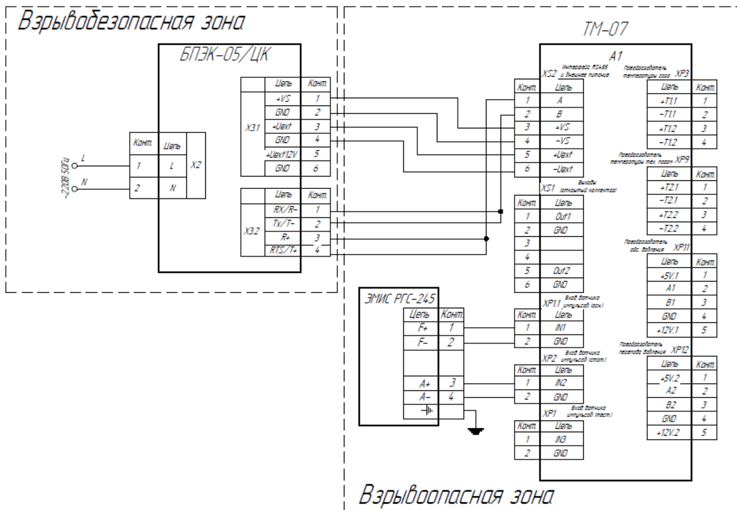
Рисунок В.5 – Схема подключения комплекса учета газа исполнения ЭМИС-ЭСКО 2230-Р-БК, где: ЭМИС-РГС245 – счетчик газа с видом взрывозащиты Exi; TM-07 – Контроллер (в комплекте ДД - датчик давления; ДТ - датчик температуры; ДТ окр.ср. - ДТ окружающей среды (по запросу), ДПД – датчик перепада давления (по запросу); БПЭК - Цифровой коммуникационный блок.
