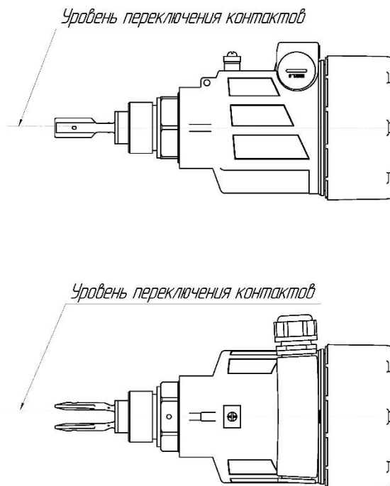
Рисунок 2.5 - Горизонтальный монтаж сигнализатора
