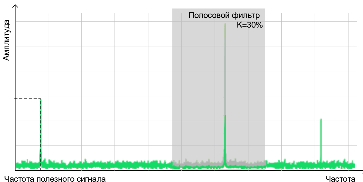
Рисунок 9.13. Полосовой фильтр
