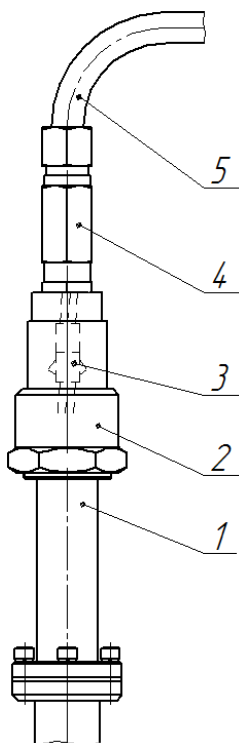
Рисунок 6.2. Разъёмное дистанционное исполнение
