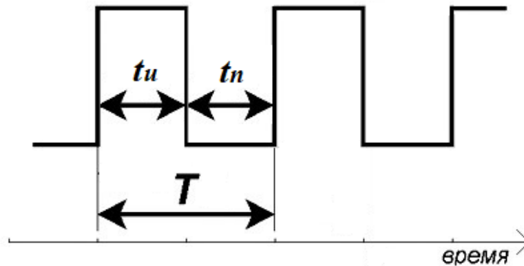
Рисунок 7.3 – Сигнал на частотно-импульсном выходе при t_i = t_p
