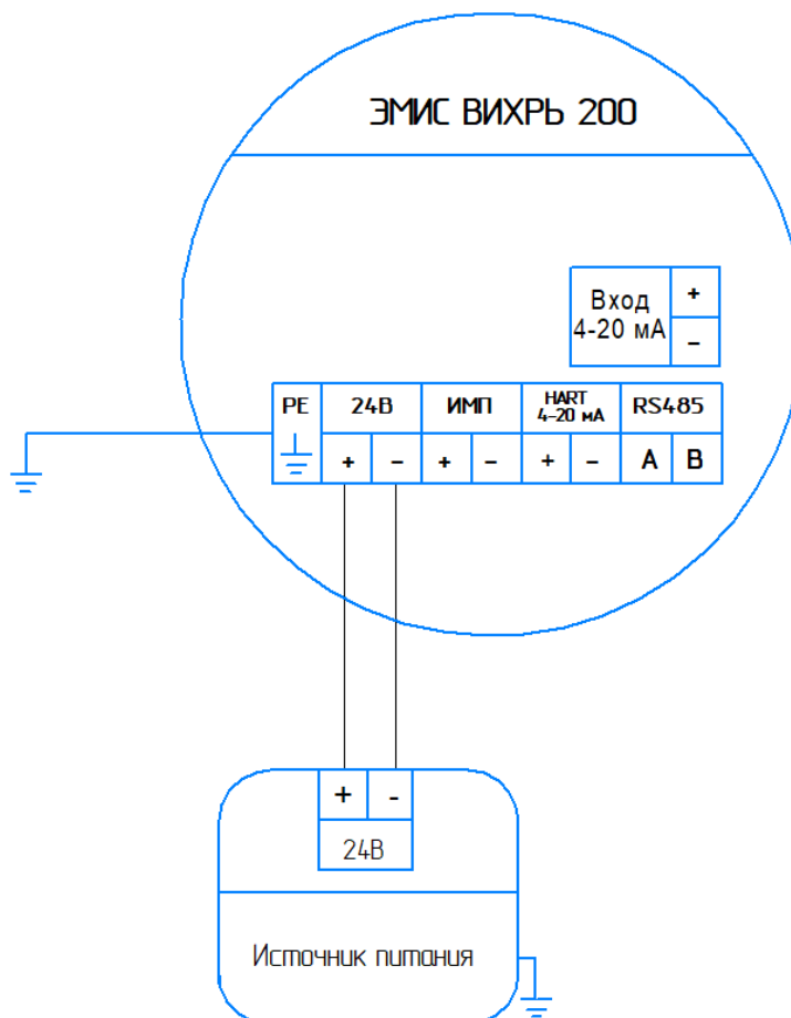
Рисунок 8.4. Схема подключения питания
