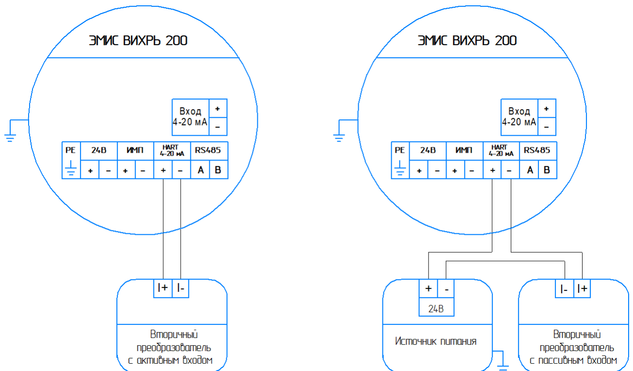
Рисунок 8.7. Схема подключения токового выхода 4-20 мА электронного блока к вторичному преобразователю с активным (слева) и пассивным (справа) токовым входом
