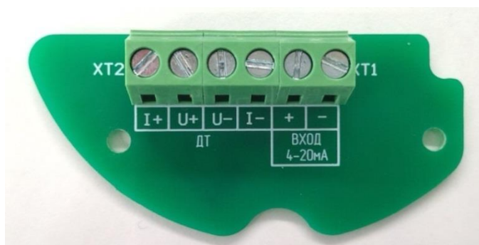
Рисунок 8.2 – Плата коммутации для подключения датчика давления и датчика температуры
