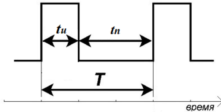
Рисунок 7.2 – Сигнал на частотно-импульсном выходе при t_i < t_p
