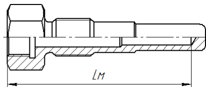
Lm гильз для термопреобразователя с неподвижным штуцером
