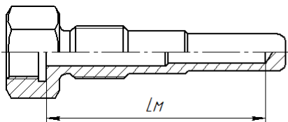
Lm гильз для термопреобразователя с подвижным штуцером
