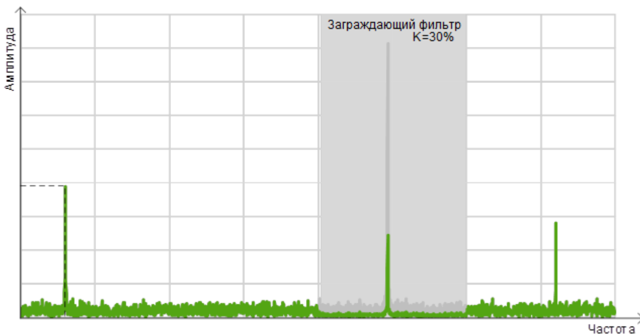
Рисунок 9.7 – Заграждающий фильтр
