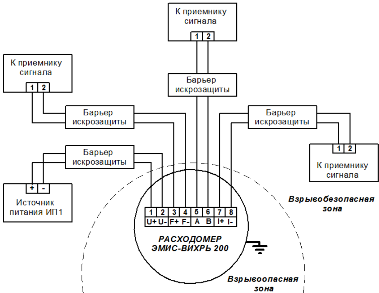
Рисунок 8.12 – Схема подключения преобразователей взрывозащищенных исполнений ExB, ExC, ExiaB, ExiaC, PVI, PO с использованием барьеров искрозащиты
