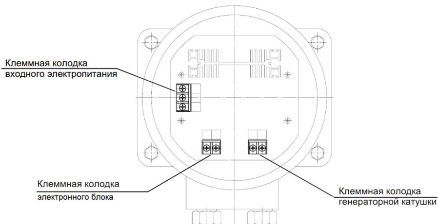
Рисунок 5.4. Усилитель.
