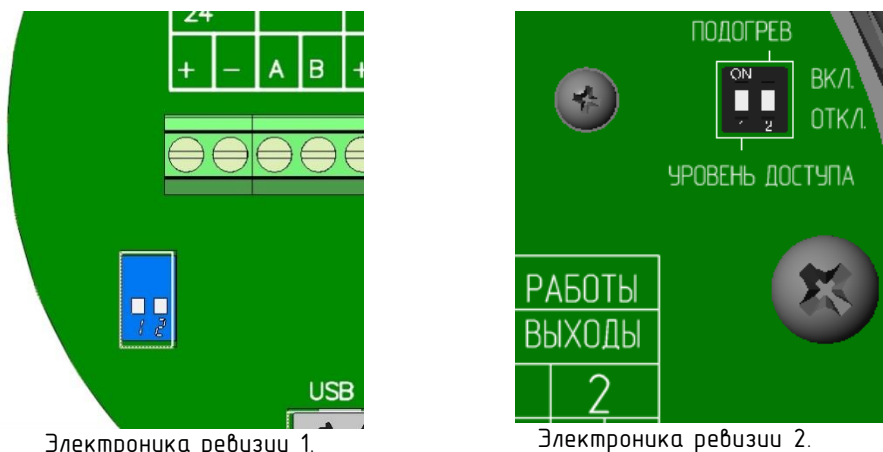
Рисунок 6.1. Переключатель уровня доступа SW1.
