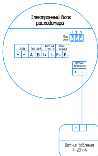
Рисунок 5.12. Схема подключения датчика давления.
