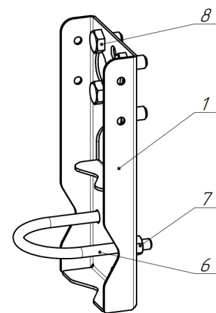
Рисунок Е.2 – Кронштейн прямой в комплекте с КМЧ
