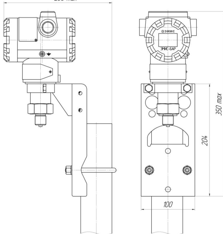
Рисунок И.1 – Монтаж датчика штуцерного исполнения на кронштейн прямой на трубе
