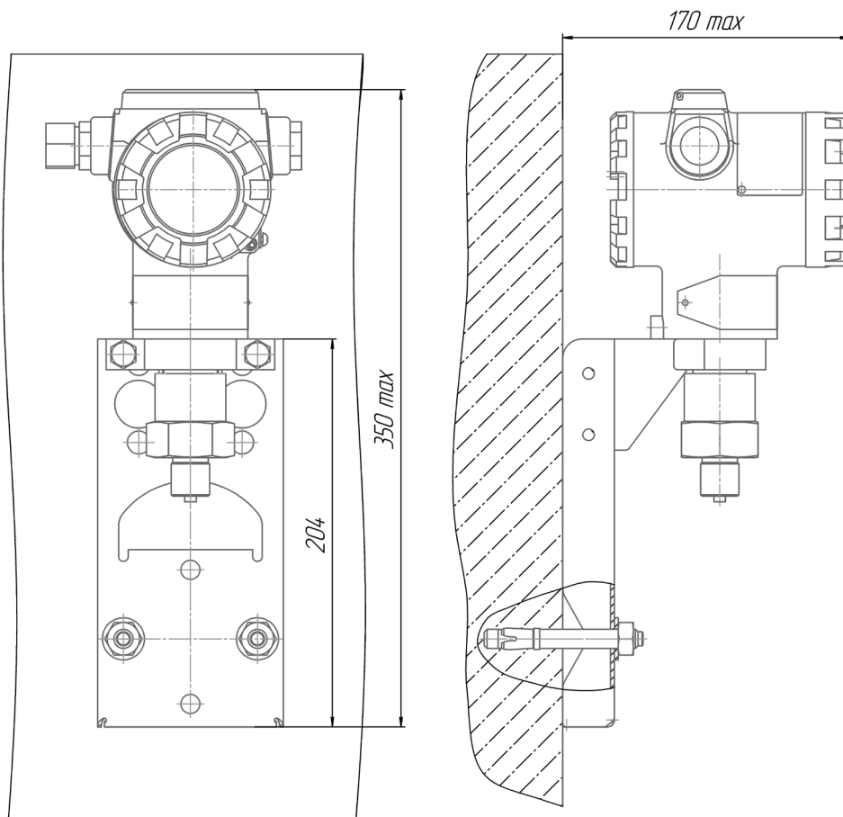
Рисунок И.1.1 – Монтаж датчика штыцерного исполнения на кронштейн прямой на стене
