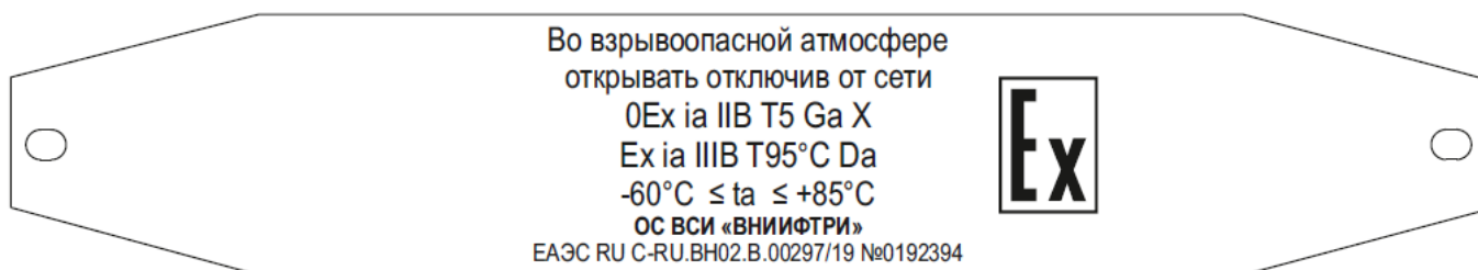
Рисунок 2.4.2 – Пример таблички для датчика взрывозащищенного исполнения
