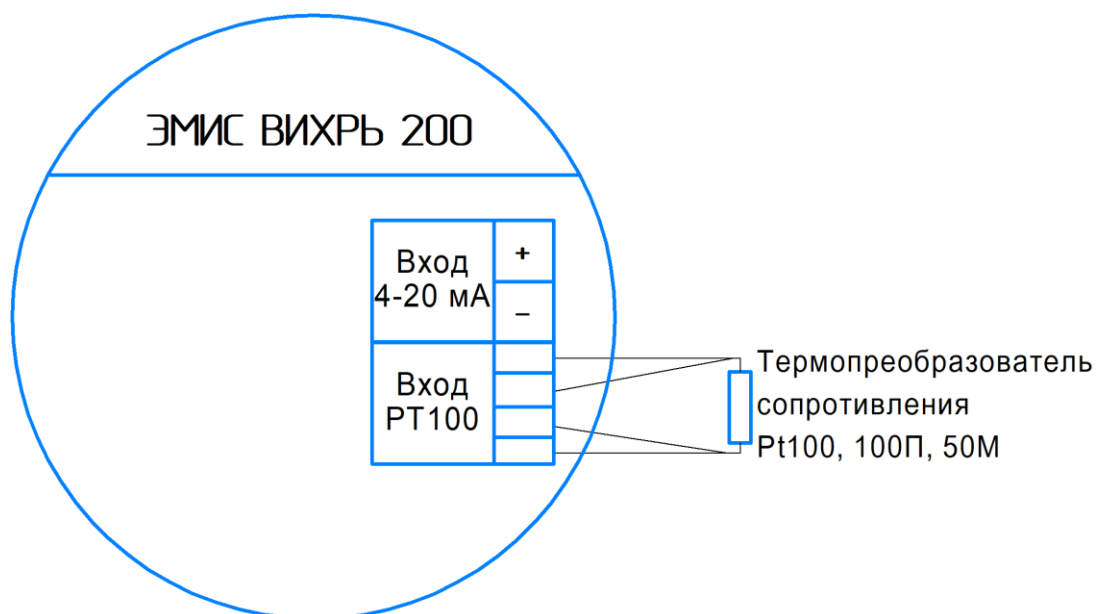
Рисунок 8.10 - Схема подключения термометра сопротивления к электронному блоку
