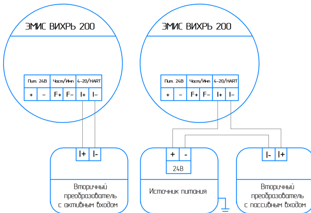
Рисунок 8.6 - Схема подключения токового выхода 4-20 мА электронного блока к вторичному преобразователю с активным (слева) и пассивным (справа) токовым входом
