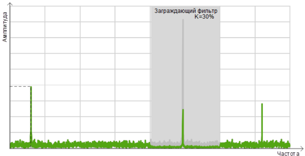
Рисунок 9.7 – Заграждающий фильтр
