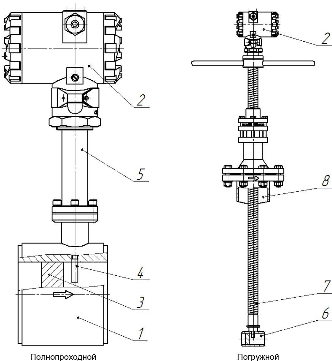
Рисунок 3.1 – Устройство расходомеров
