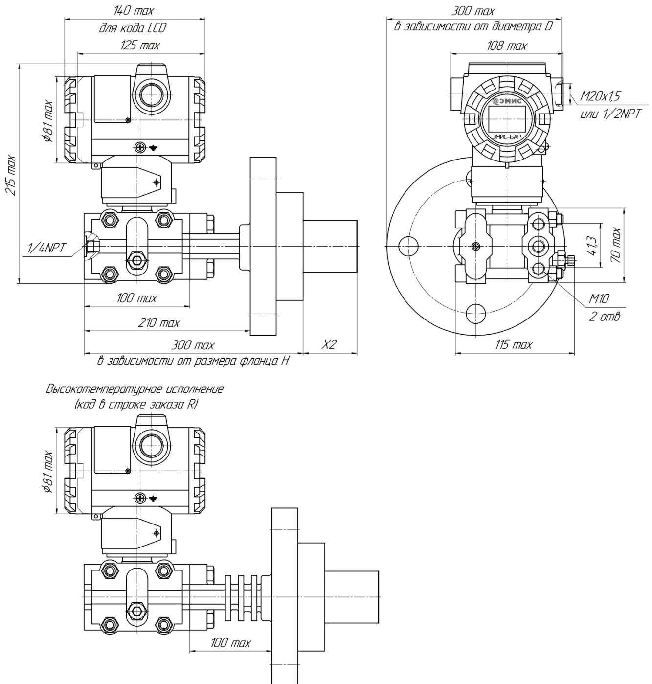
Рисунок Д.6 – Габаритные и присоединительные размеры специального фланцевого исполнения датчиков давления ЭМИС–БАР 164.
