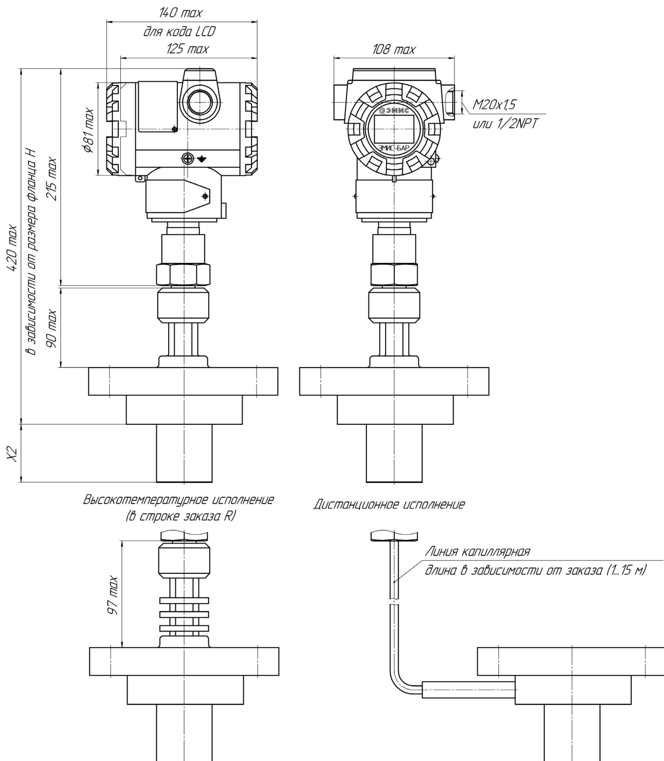
Рисунок Д.8 – Габаритные и присоединительные размеры специального фланцевого исполнения датчиков давления ЭМИС-БАР 174 и 176.
