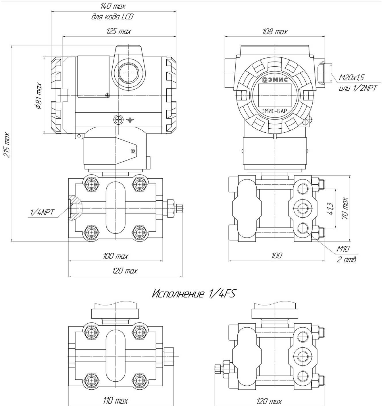
Рисунок Д.2 – Габаритные и присоединительные размеры фланцевого исполнения (DIN 19213) датчиков давления ЭМИС-БАР 105 (кроме диапазонов HS) и 133
