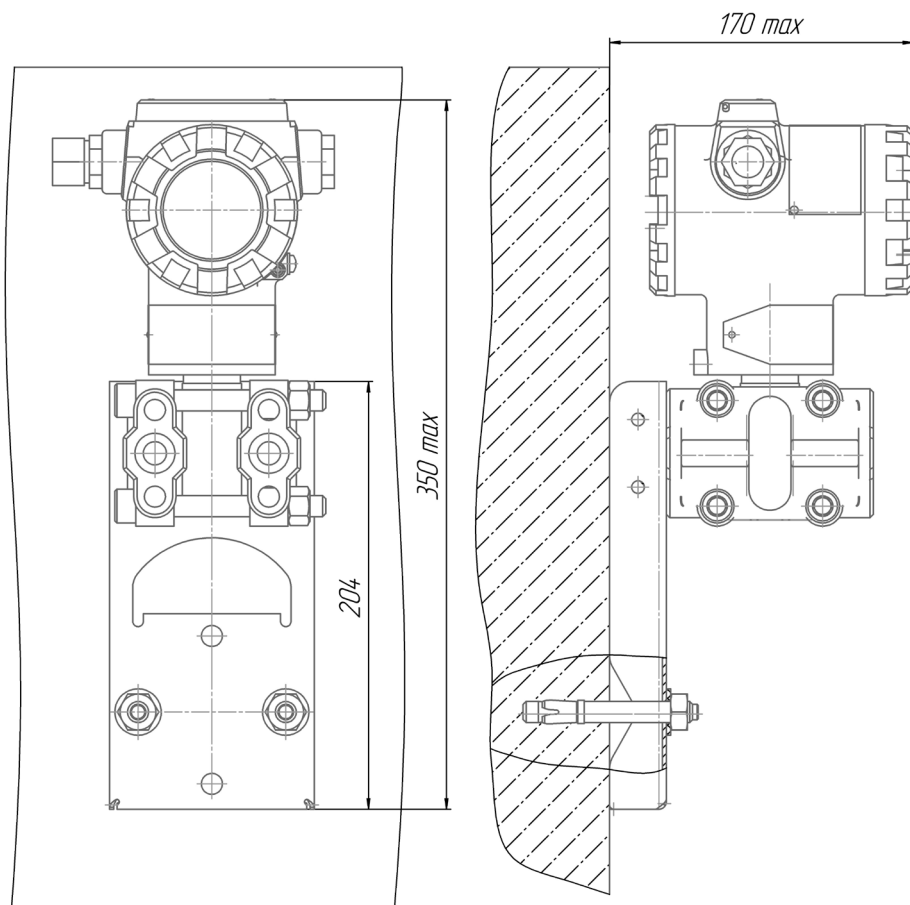
Рисунок И.2.1 – Вариант монтажа датчика фланцевого исполнения на кронштейн прямой на стене
