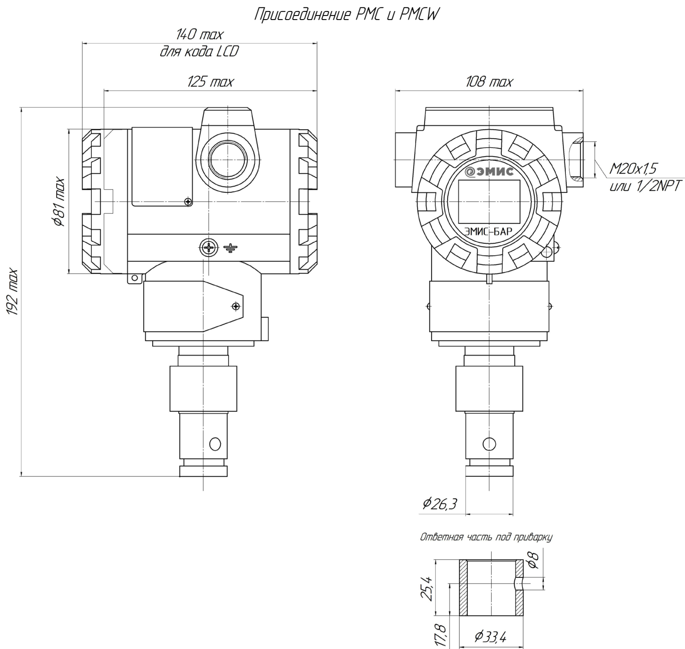
Рисунок Д.4.1 – Габаритные и присоединительные размеры штуцерного исполнения с открытой мембраной (присоединение PMS, PMSW (Minibolt, 1 дюйм)) датчиков давления ЭМИС–БАР 113
