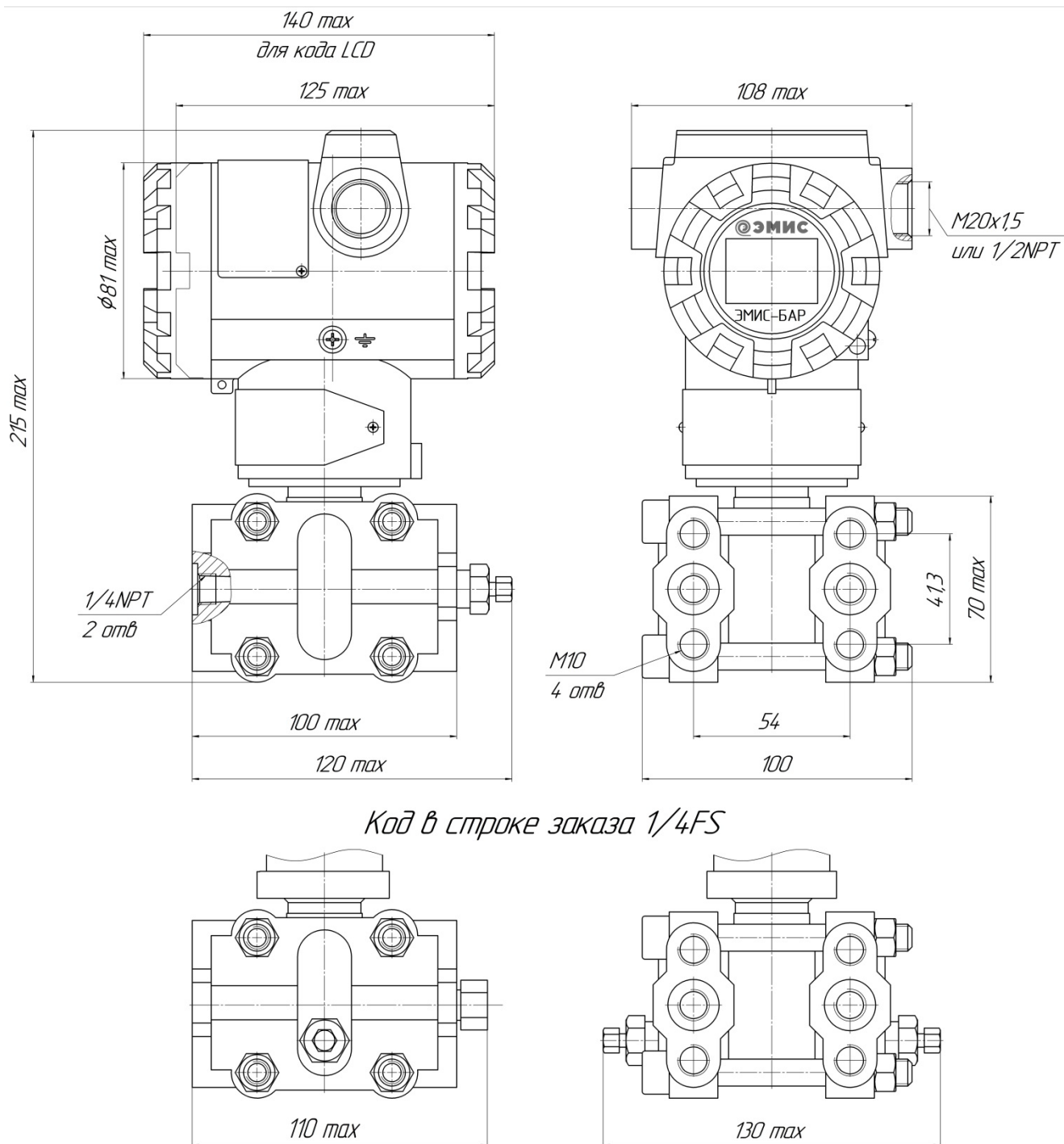
Рисунок Д.3 – Габаритные и присоединительные размеры фланцевого исполнения (DIN 19213) датчиков давления ЭМИС-БАР 143, 153, 193, 105 (с диапазонами Нs)
