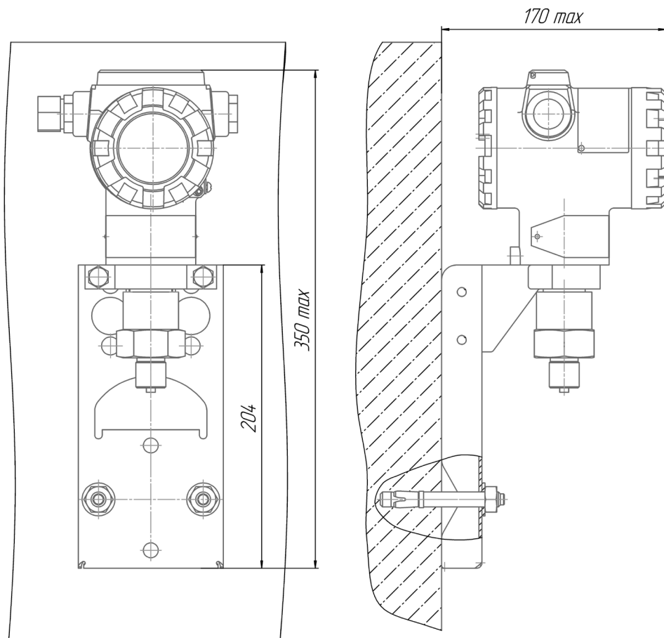
Рисунок И.1.1 – Вариант монтажа датчика штуцерного исполнения на кронштейн прямой на стене
