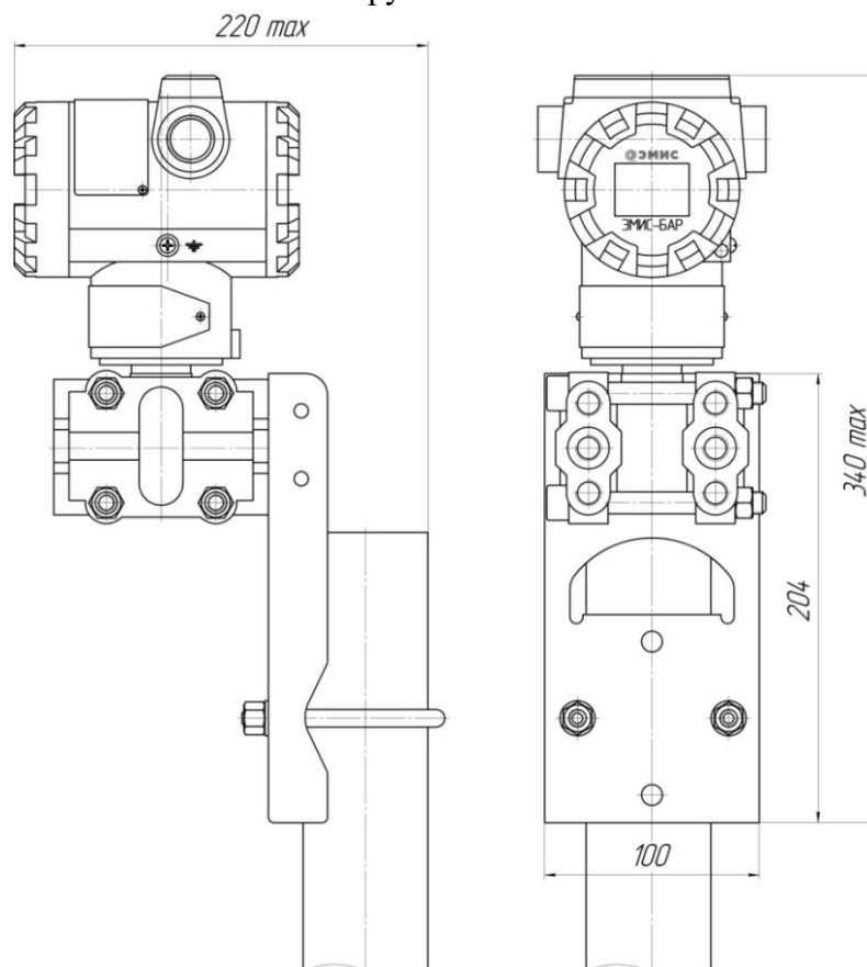
Рисунок И.2 – Вариант монтажа датчика фланцевого исполнения на кронштейн прямой на трубе
