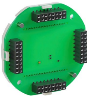
а. Плата индикатора. Вид сзади.
