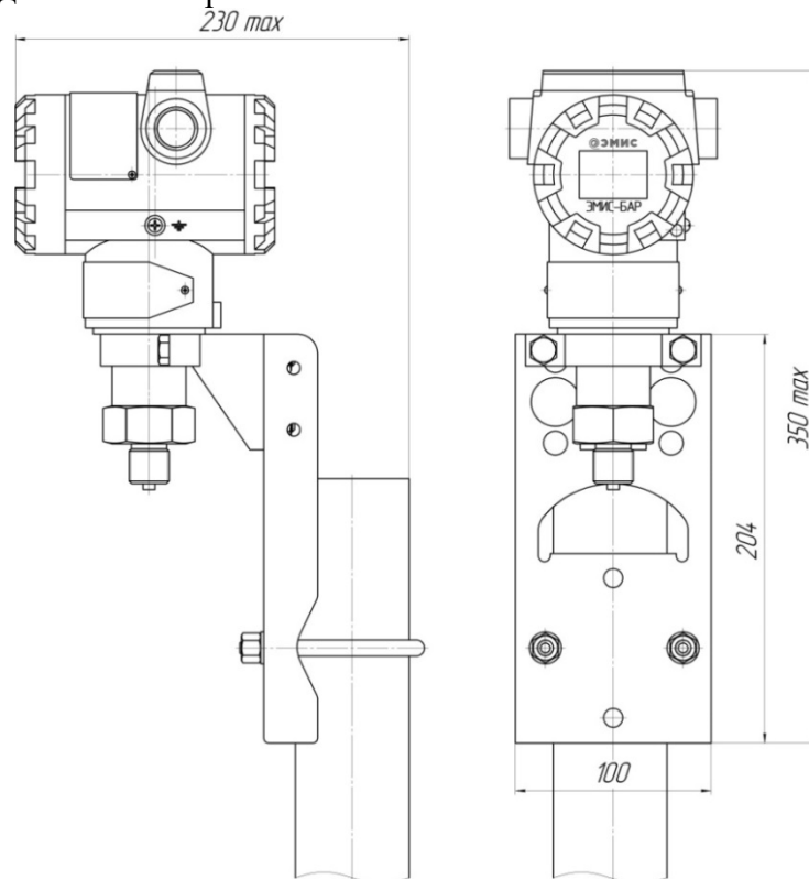
Рисунок И.1 – Вариант монтажа датчика штуцерного исполнения на кронштейн прямой на трубе
