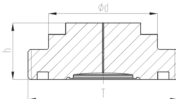
Габаритные и присоединительные размеры штуцера молочной гайки SMS1145
