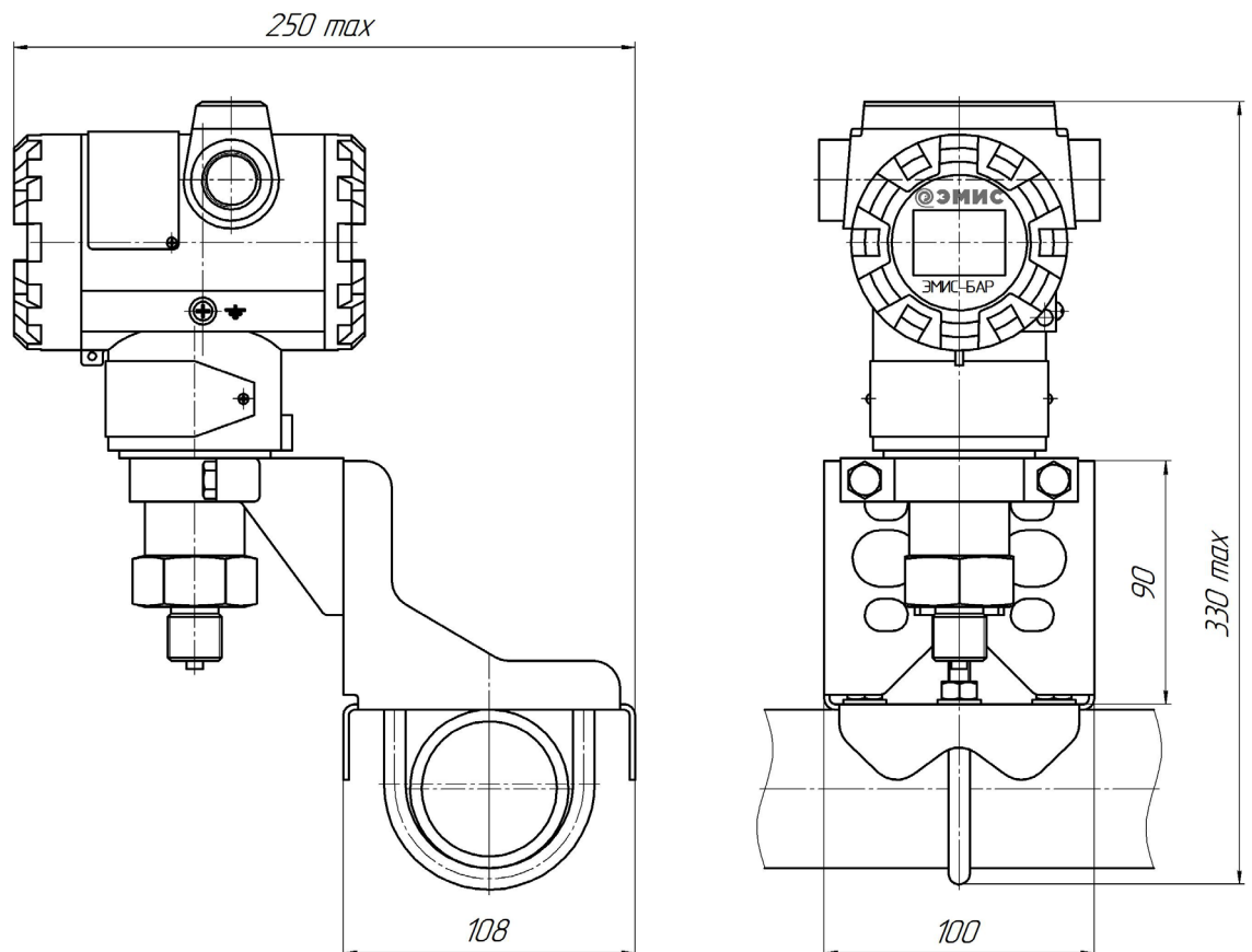
Рисунок И.3 – Вариант монтажа датчика штуцерного исполнения на кронштейн угловой (код материала «CS» и «S»)
